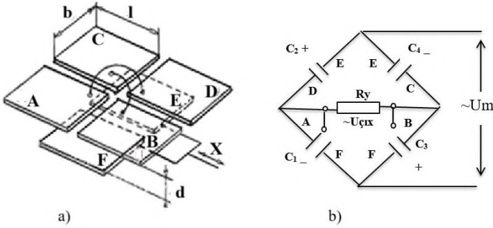
Şəkil 2.1. Tutum yerdəyişmə çeviricisi
