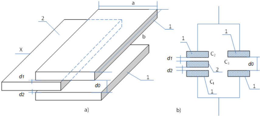
Şəkil 3.2. TV-in konstruksiyası (a) və ekvivalent sxemi (b)
