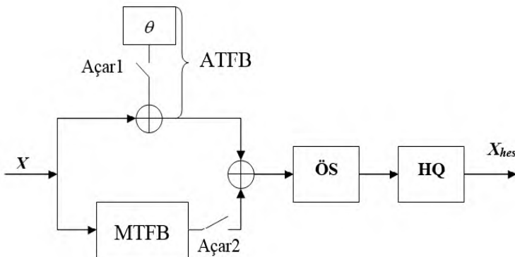
Şəkil 4.1. Testləşdirilmiş İÖS-in struktur sxemi
