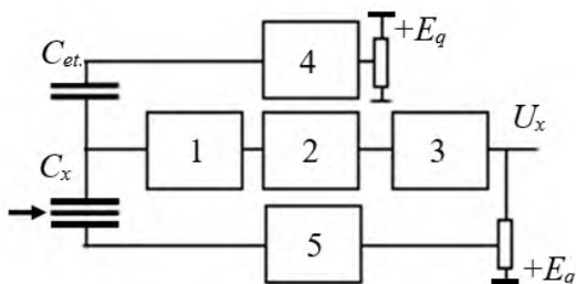
Şəkil 3.5. Böyük yerdəyişmələrin yüksək dəqiqliklə ölçmə qurğusu
