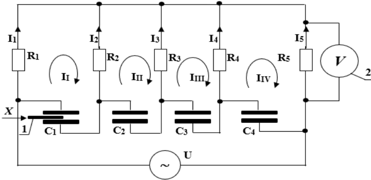
Şək. 3.3. Böyük xətti yerdəyişməli tutum vericisinin sxemi
