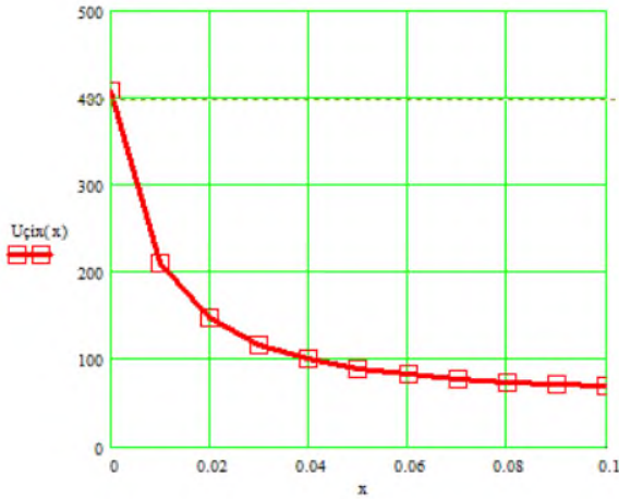
Şekil 3.4 b. U_{çix}(x)=f(x) asılılığı
