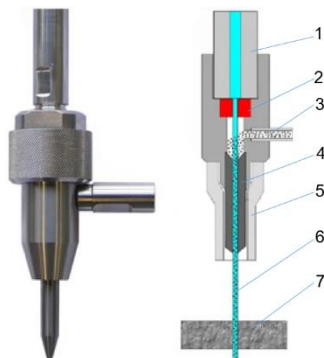
Şəkil 1. Hidroabrazivlə kəsmə sxemi
