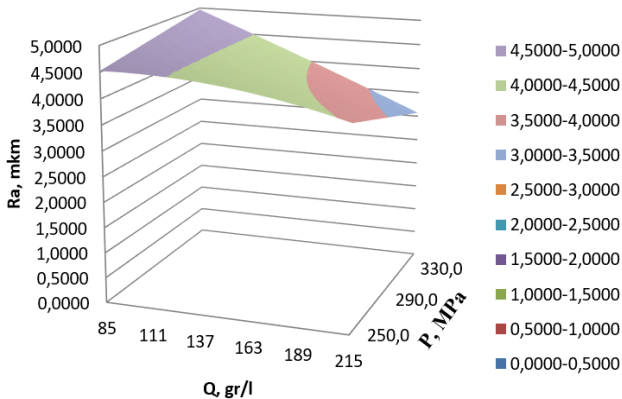
Qrafik 1. R_a –nın massiv üzrə verişdən asılı olaraq dəyişməsi
