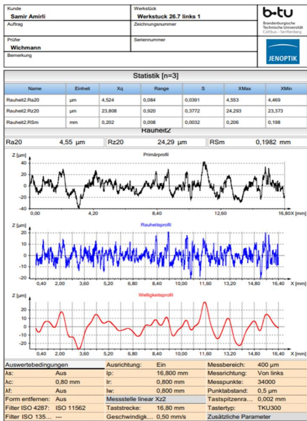
Şəkil 5. Hidroabrazivlə kəsilmiş pəstahın səthinin sol tərəfdən kələ-kötürlüyünün və dalğavariliyinin JENOPTİK cihazı vasitəsilə ölçülməsinin nəticələri
