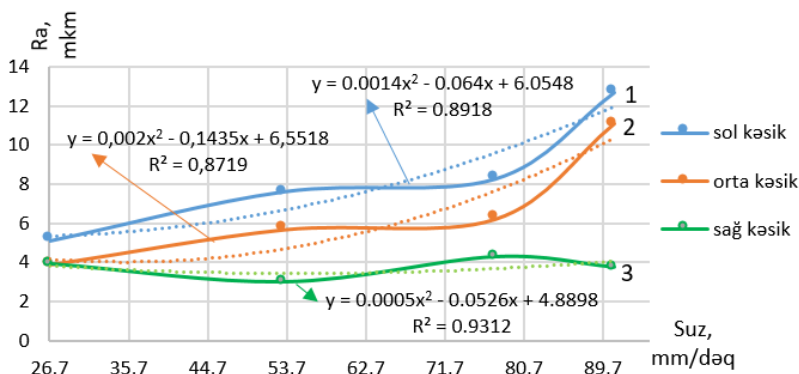
Qrafik 3. Uzununa veriş hərəkətindən asılı olaraq müxtəlif en kəsiklər üzrə kələ-kötürlüyün orta hündürlüyünün ( R_a )-təcrübədən alınma ayrılırları
