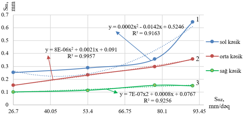
Qrafik 5. Kələ-kötürlüyün orta addımının uzununa verişdən asılı olaraq dəyişmə ayrılırları
