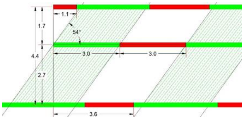
Şəkil 10. Akademik Zərifə Əliyeva küçəsində qurulmuş əlaqələndirilmiş nizamlaşma qrafiki
