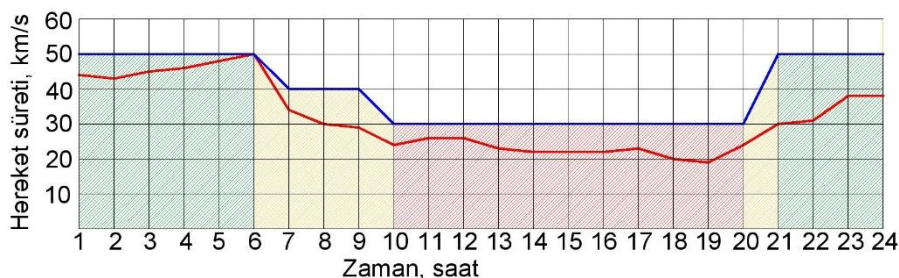
Şəkil 11. “Yaşıl dalğa” rejiminin adaptiv tənzimlənməsi ilə nəqliyyat axının vəziyyəti
